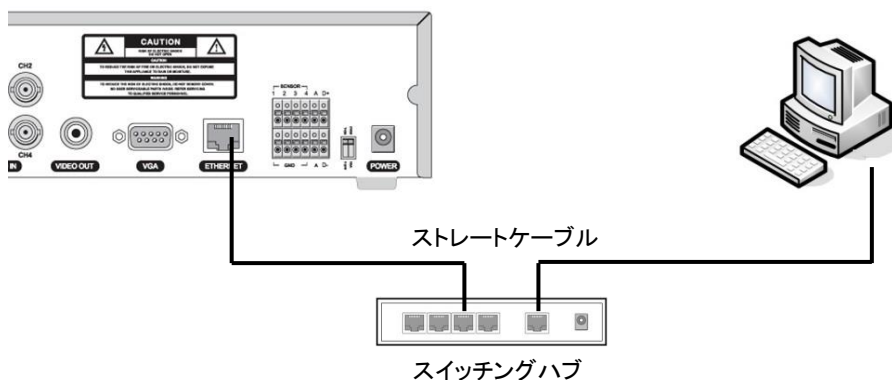
スイッチングハブ
