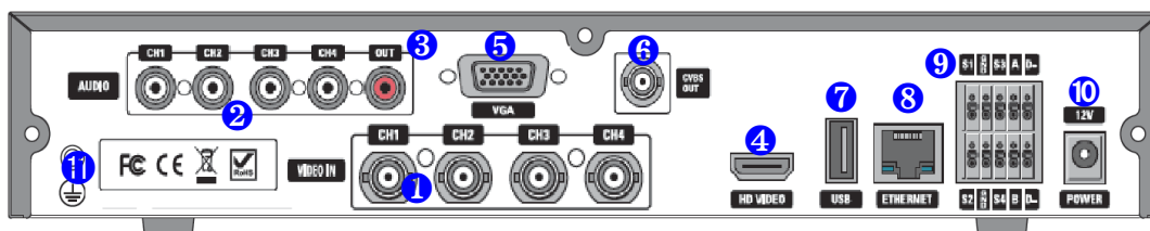
背面端子の説明
