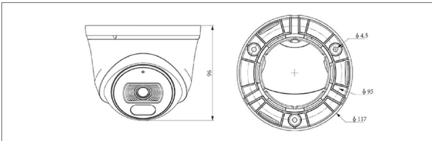
外観図面
